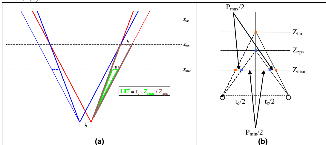
Figura 11.6 – a) Cálculo do HIT. b) Cálculo de t_c dado Z_{zps} .
