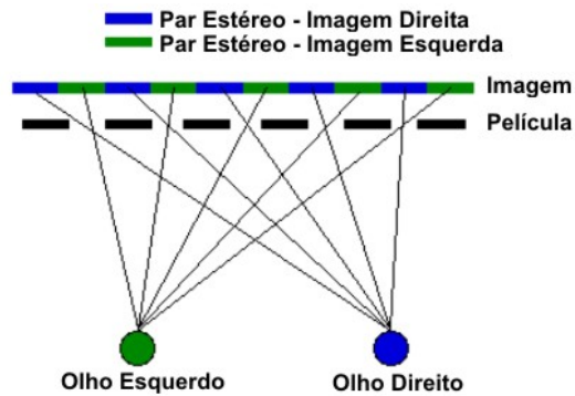
Figura 11.19 – Display Autoestereoscópico.
