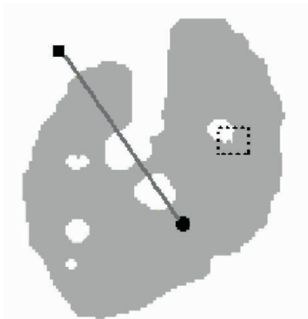
Figura 2. A componente conexa em cinza, o fundo em branco, um ponto qualquer pertencente à componente é o círculo preto, um ponto qualquer não pertencente à componente conexa é o quadrado preto.
